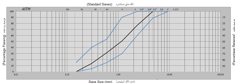
ب) نمودار دانه بندی ریزدانه (ماسه)
