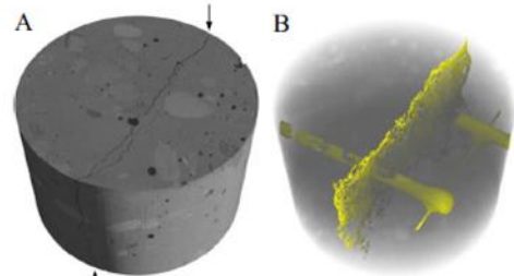
شکل ۲ شکستن شیشه های محتوی پلی اورتان و خروج چسب از داخل آن ها و پرکردن ترک های ایجاد شده ناشی از خمش. (Tittel boom et al., 2017)
