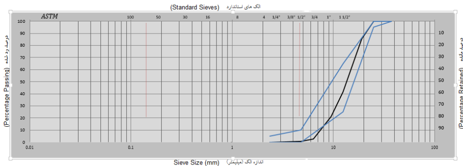
الف) نمودار دانه بندی درشت دانه (شن)
