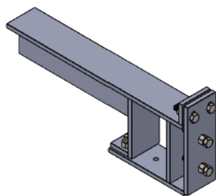
شکل ۶ نمایی از دستک و ابعاد و اندازه آن ها
