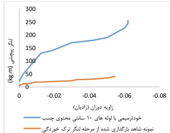
نمودار ۸ نمودار لنگر پیچشی بر حسب زاویه دوران، برای نمونه شاهد و نمونه ترمیم شده با روش خودترمیمی به کمک لوله‌های ۱۰ سانتی متری محتوی چسب
