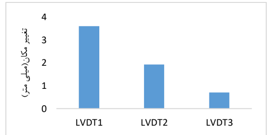
نمودار ۶ نمودار تغییر مکان LVDT های استفاده شده برای نمونه ترمیم شده با روش لوله‌های یک متری
