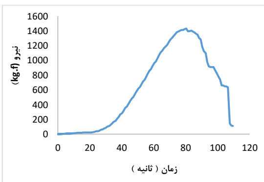
نمودار الف- نمودار نیرو بر حسب زمان برای نمونه شاهد
